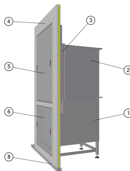
1 - Stenový nadstavec; 2 - Nadstavec TROX; 3 - Límeč; 4 - Panel hr. 60mm; 5 - Revízny poklop, 6 - Mriežka, 8 - Basic profil
