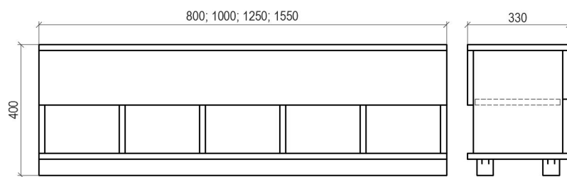
PL2 PL2 - překročná lavica obojstranná
