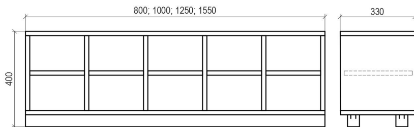
PL1 PL1 - překročná lavica jednostranná
