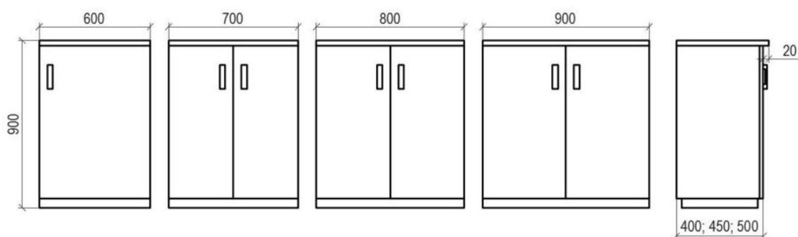
Шкаф для мойки, устанавливаемый в шлюз
