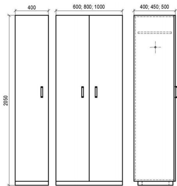
Шкаф с вешалками открытый
