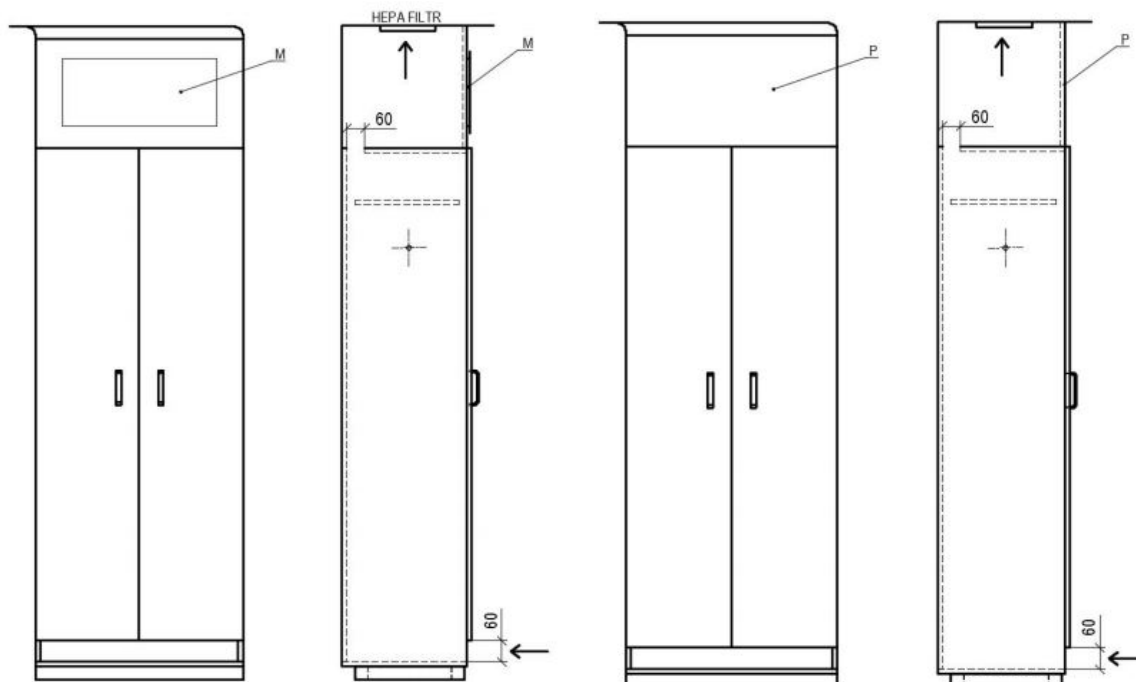
Проветриваемый шкаф с вешалками
