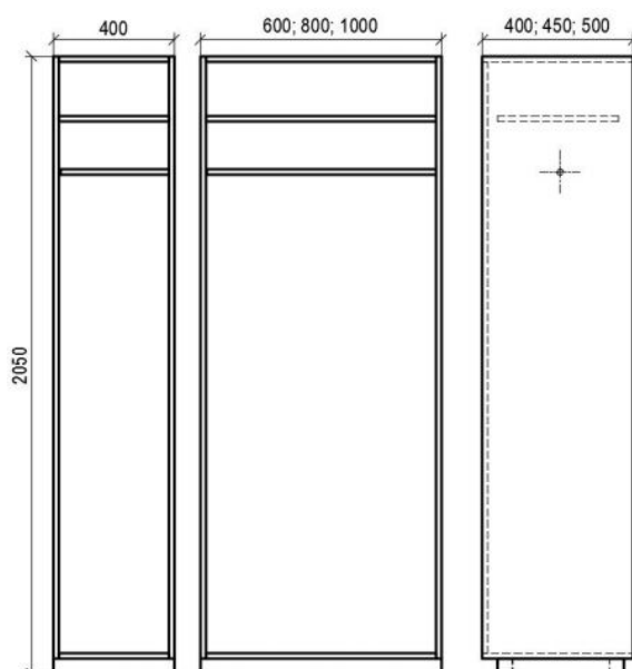
Шкаф с вешалками открытый
