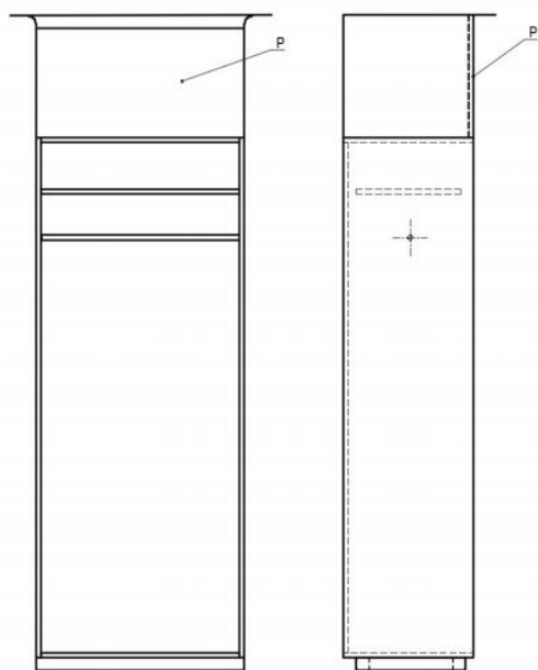
Закрытие места соединения открытого шкафа с потолком
