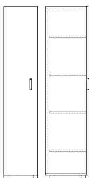
04 Policová skříň
