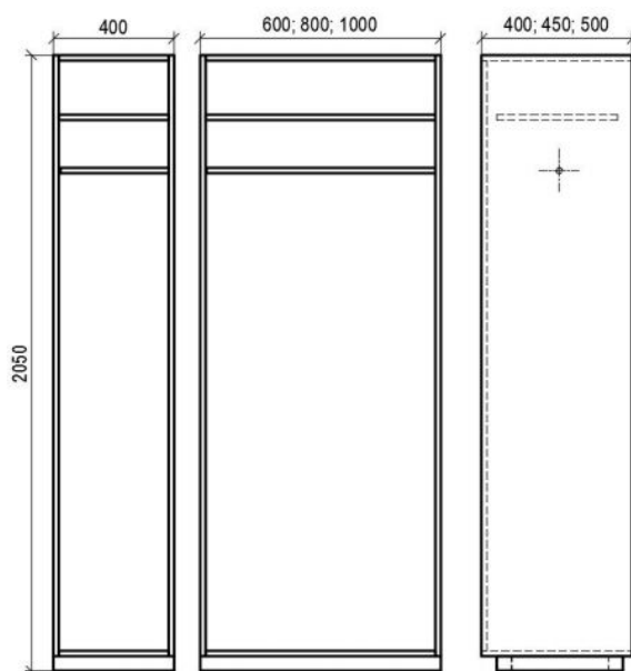
Věšáková skříň otevřená
