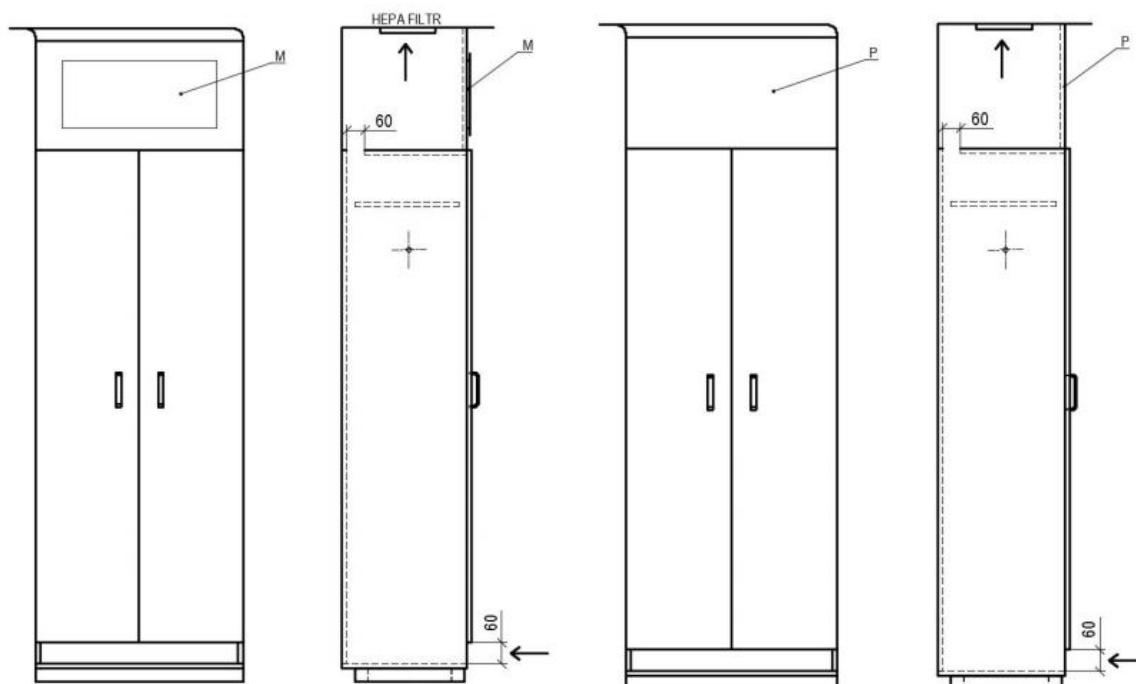
Odsávaná věšáková skříň s HEPA filtrem
