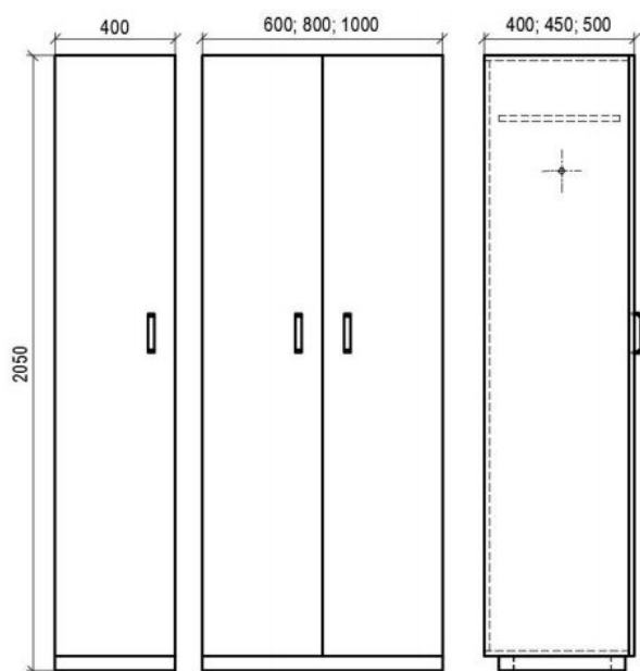
Věšáková skříň uzavřená
