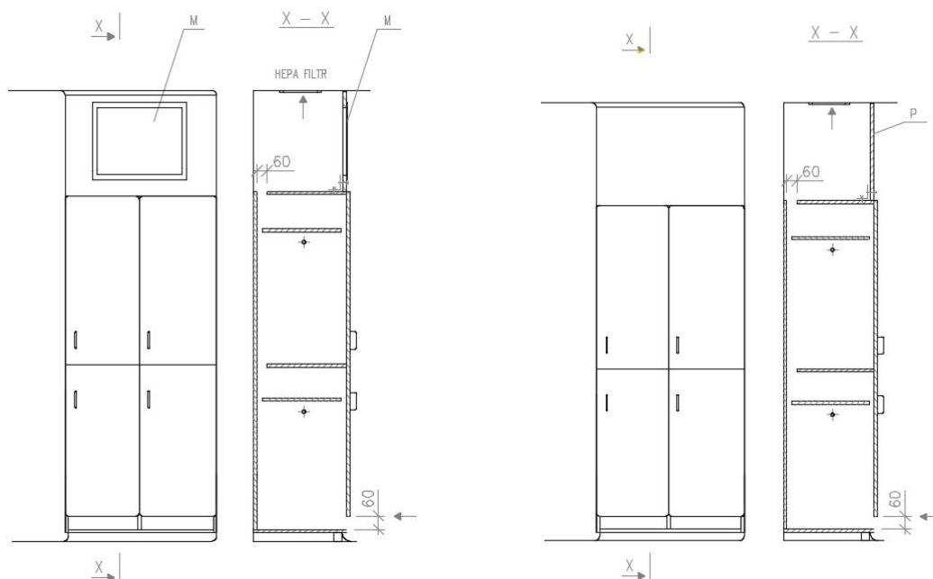
Dokrytování z lisovaných dřevotřískových desek se servisními dvířky
