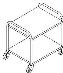
Manipulační stolek se dvěma policemi
