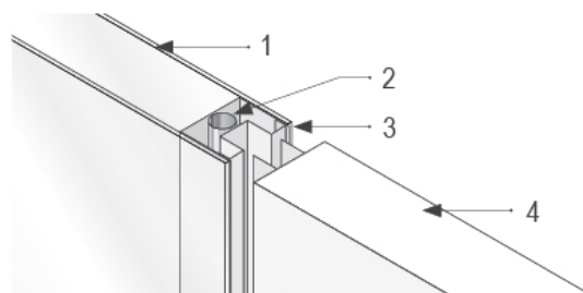
1 - Sklo; 2 - Elektroinstalační průchodka; 3 - Tmelení; 4 - Příčkový panel
