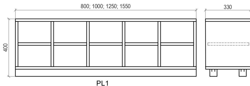
PL1 - překročná lavice jednostranná
