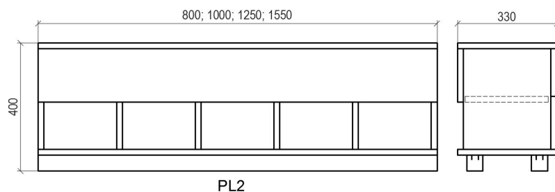
PL2 - překročná lavice oboustranná
