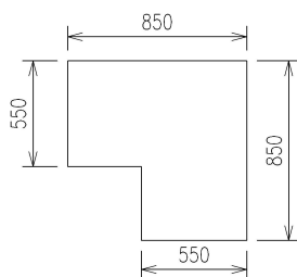
RH1 Rohová skřínka pravoúhlá - vnitřní roh
